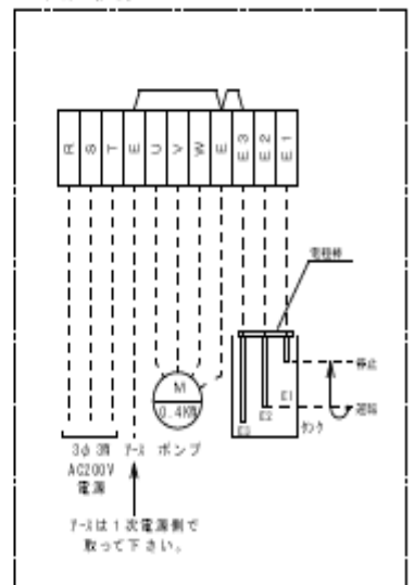
外部端子接続図
